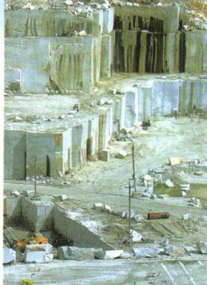
Метаморфические горные породы
