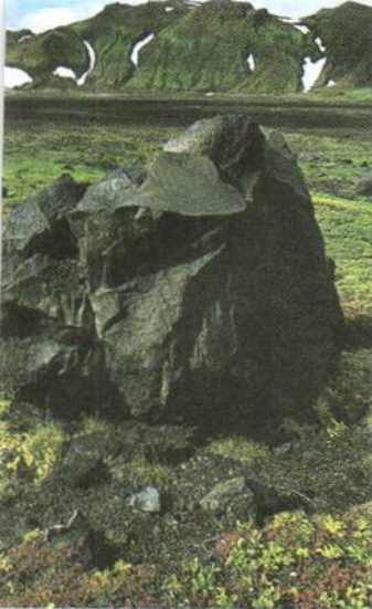
Магматические горные породы
