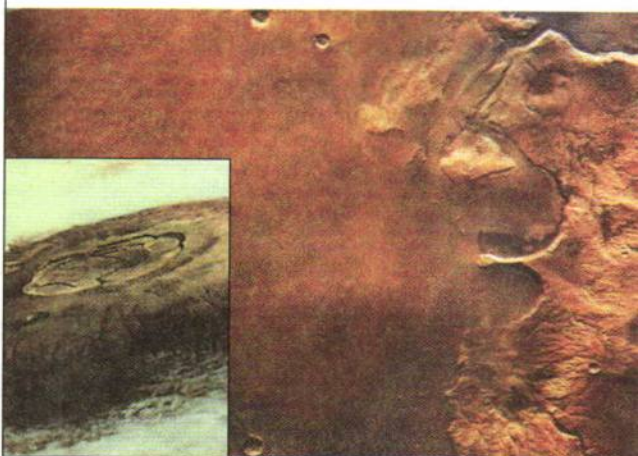
Потухший вулкан на Марсе — гора Олимп
