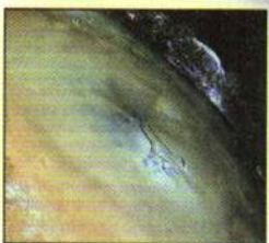
Спутник Урана — Миранда
