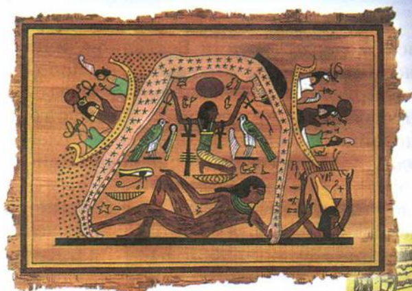
Вселенная в представлении древних египтян
